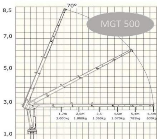
DIAGRAMA OPERACIONAL DE CARREGAMENTO E ALCANCE
